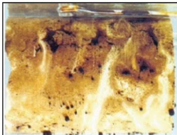
Roche-réservoir: carotte de forage imprégnée de pétrole.
