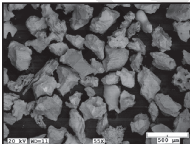
Cendres volcaniques recueillies au volcan Veniaminof (Alaska), août 2013 (500 μm équivaut à 0,5 mm). Photo : Kristi Wallace, United States Geological Survey. » https://scir.rncan.gc.ca/volcano-volcan/hazard-risque-fr.php
