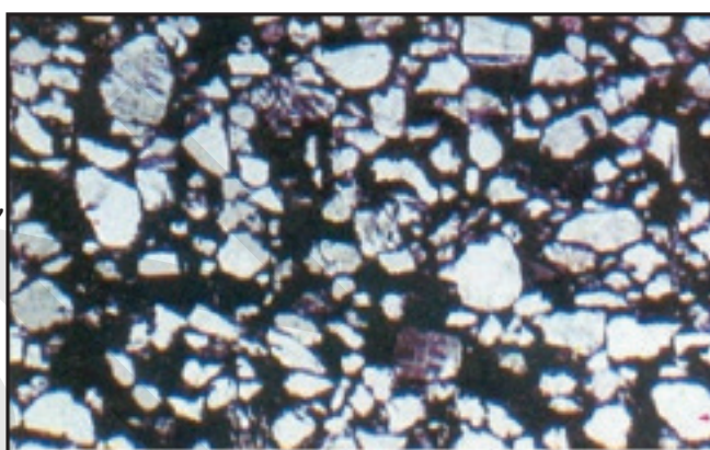
lame mince de roche- réservoir avec grains de quarts imprégnés de pétrole.
